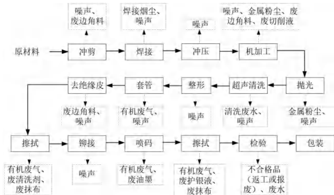
图 2-7 软连接生产工艺流程图
