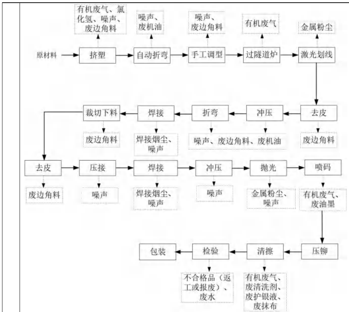
图 2-13 挤塑母排生产工艺流程图
