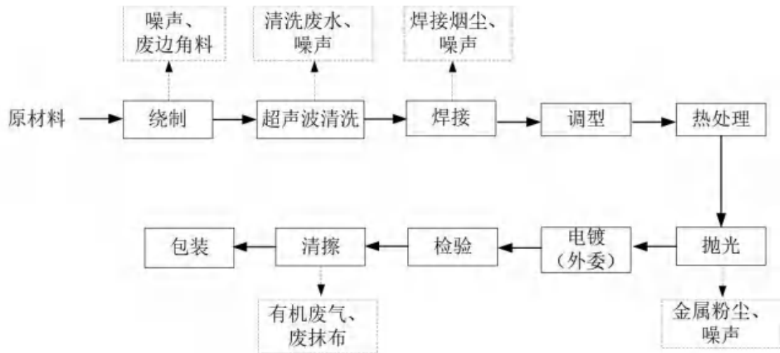
图 2-11 弹簧触指生产工艺流程图
