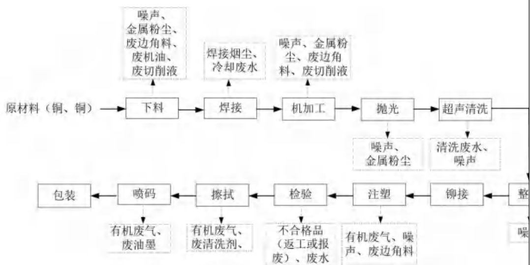
图 2-16 注塑母排生产工艺流程图
