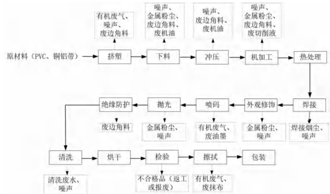
图 2-10 编织线生产工艺流程图
