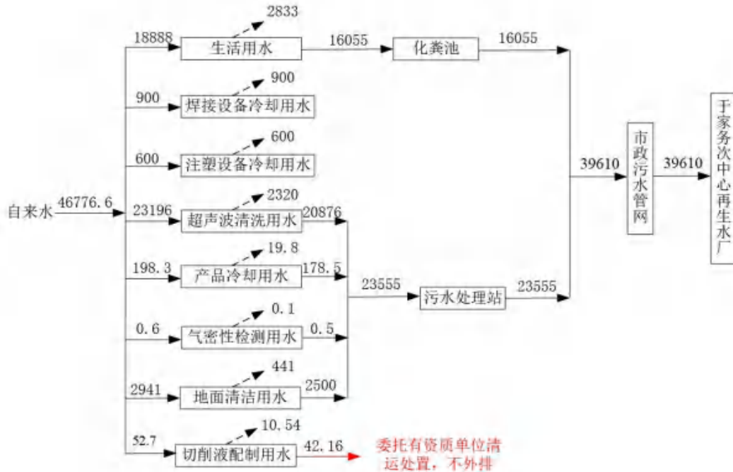
2-6 全厂水平衡图 m^3/a
