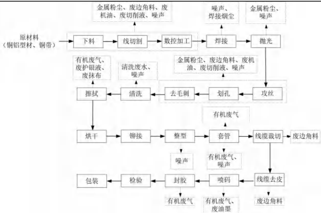
图 2-15 柔性快插生产工艺流程图
