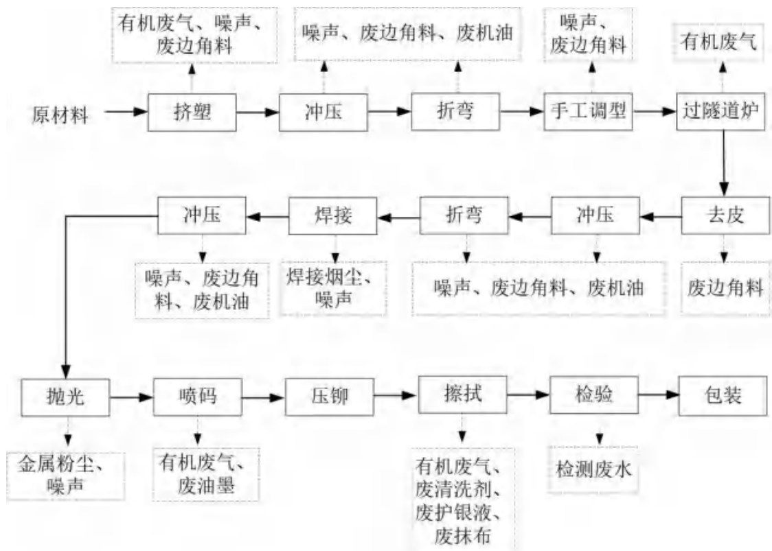
图 2-9 软母排排生产工艺流程图
