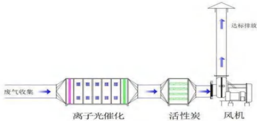
图 4-1 UV 光氧+活性炭处理工艺流程简图
