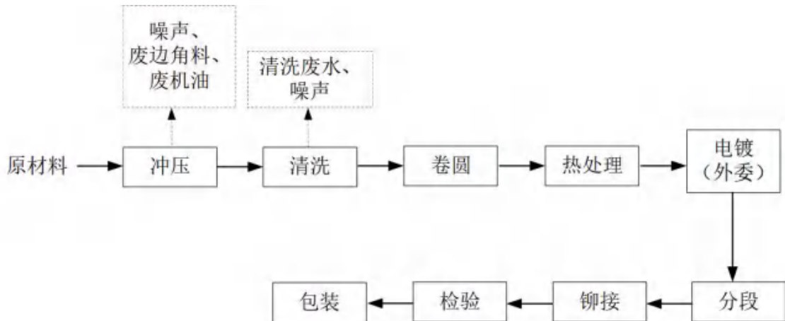
图 2-14 表带触指生产工艺流程图
