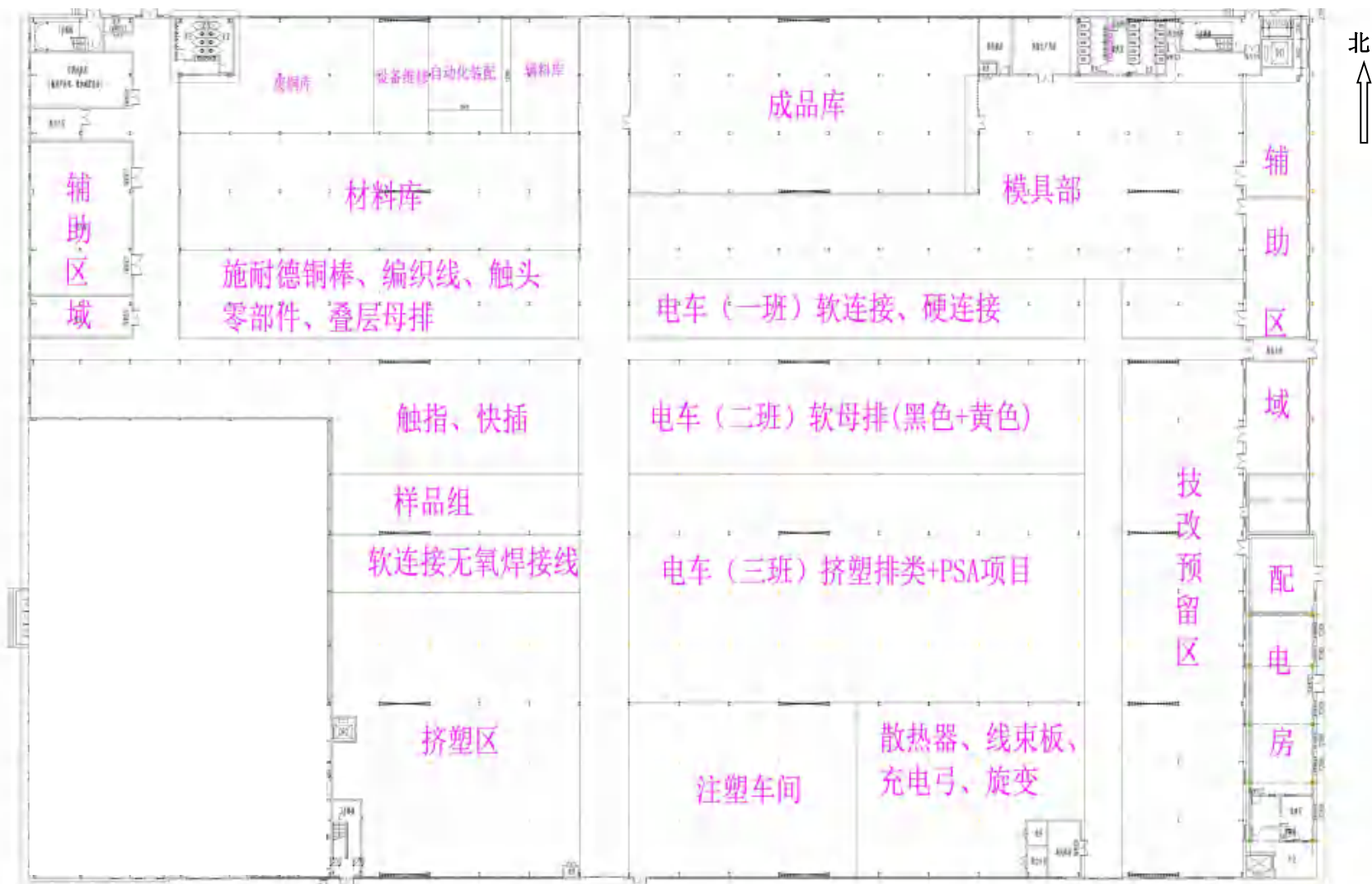
附图3 建设项目北车间平面布置图
