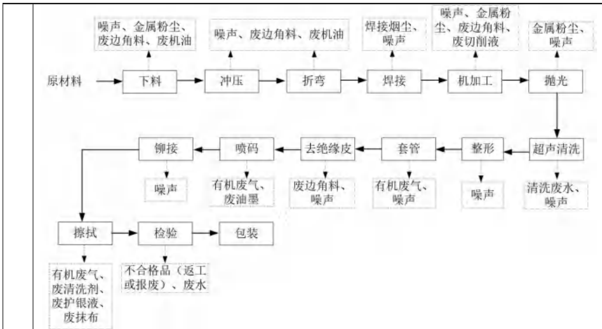
图 2-8 硬连接、触头零部件、叠层母排生产工艺流程图
