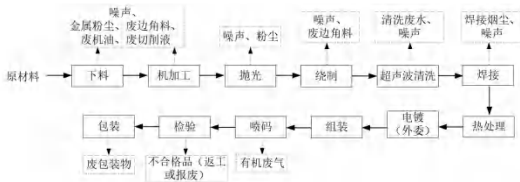
图 2-12 铝座触指、充电弓生产工艺流程图
