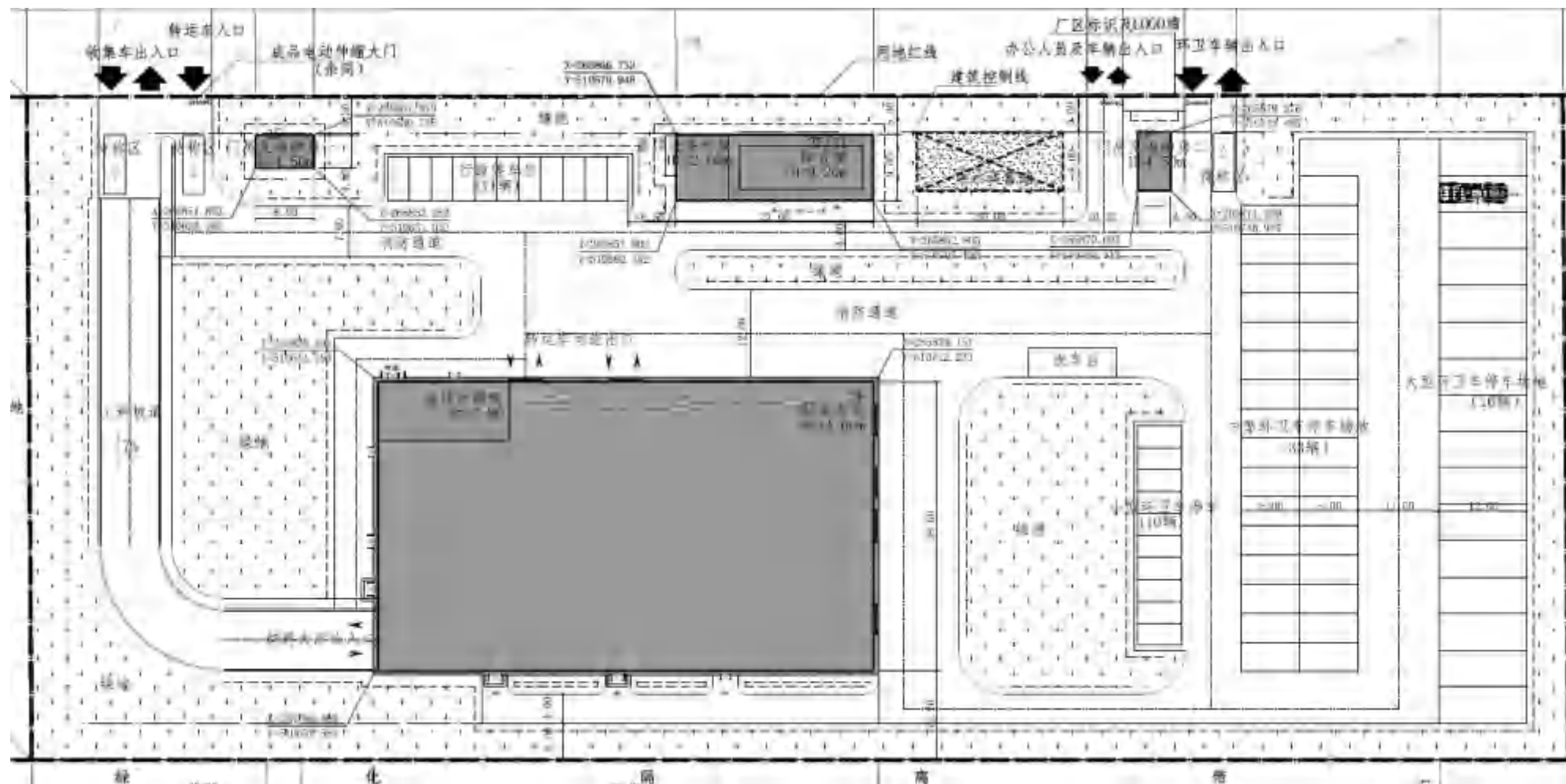
附图3 本项目总平面布置图
