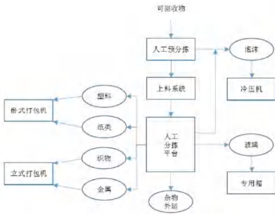
图 2.2-3 本项目可回收物中转工艺流程及产污节点图
