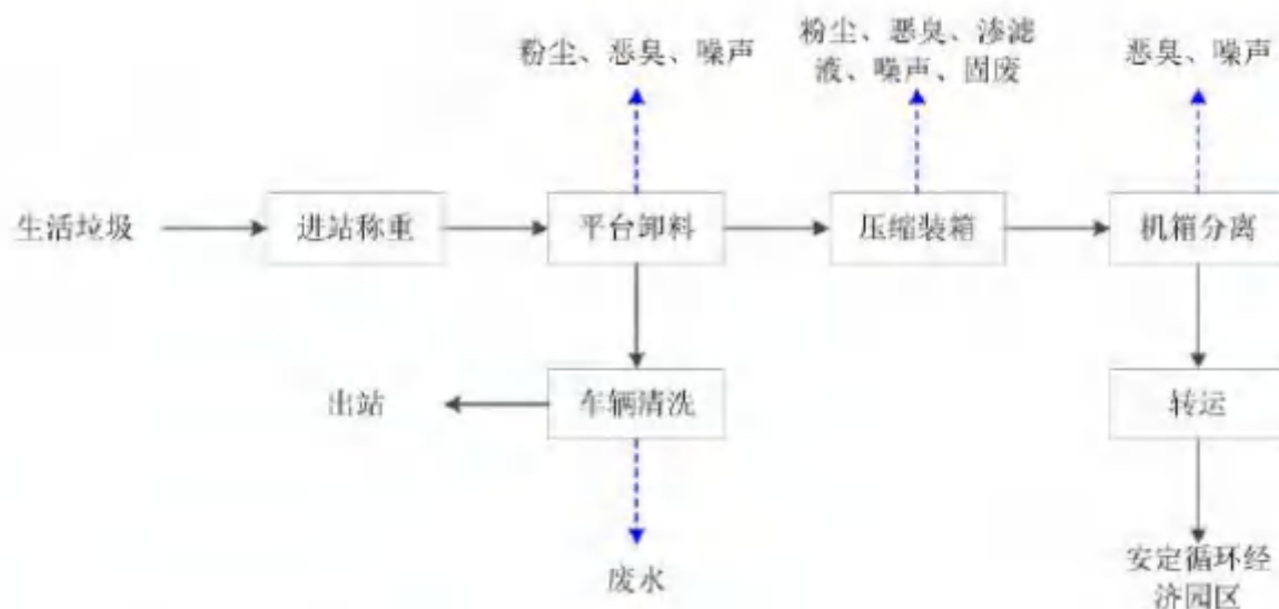
图 2.2-2 本项目生活垃圾转运工艺流程图
