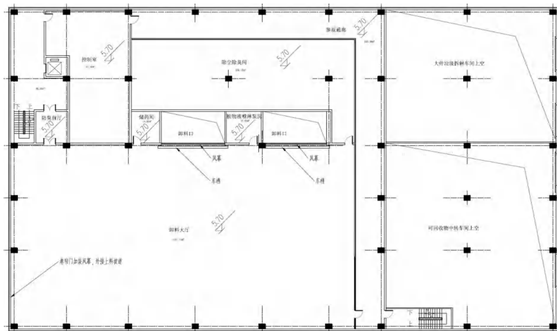
附图 5 转运车间楼二层平面布置图
