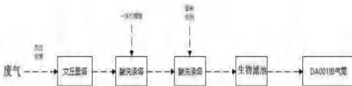
图 4.1-1 本项目废气处理工艺图
